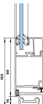
Helgerade dörrblad, utåtgående med anslagstättning
