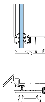
Helgerade dörrblad, inåtgående med anslagstättning
