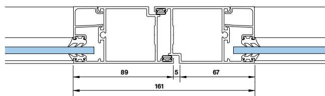
Mötesdörrar, smalprofil
