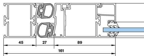
Klämfri bakkant, gummlister
