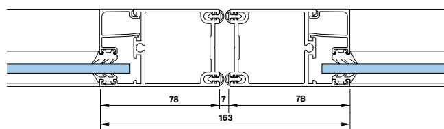
Pardörrar utan anslag, smalprofil
