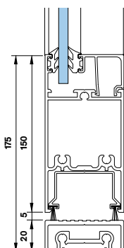
Sockelprofil med borsttätning
