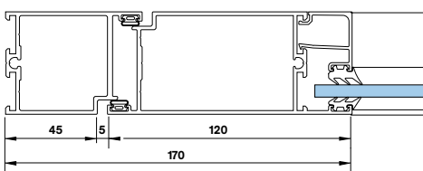
Modulprofil
