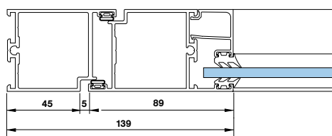
Smalprofil
