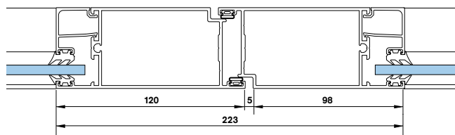
Mötesdörrar, modulprofil
