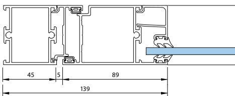
Smalprofil med bytbart anslag
