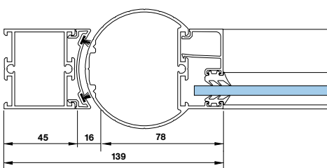
Klämfri bakkant, rundad aluminiumprofil
